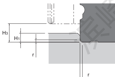
带防尘盖的LM滑块侧面图
