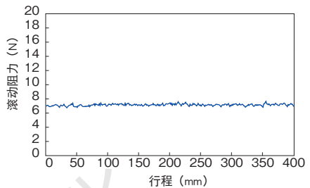
SHS25LV型的滚动阻力变动数据 (进给速度：10mm/sec)
