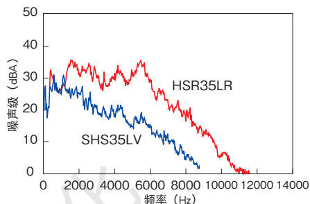
SHS35LV型—HSR35LR型的噪声级比较 (速度为50m/min时)
