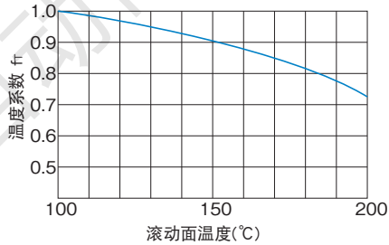
图9 温度系数 (f T )
