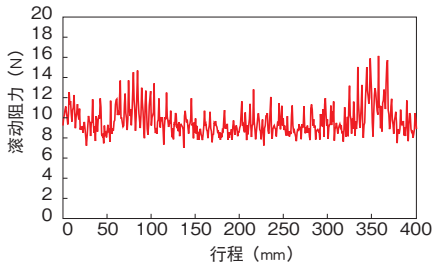
HSR25LR型的滚动阻力变动数据 (进给速度：10mm/sec)
