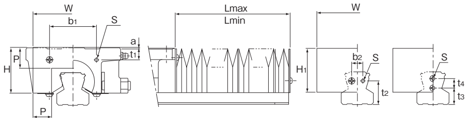
NSR30~70TBC型 NSR20、25TBC型
