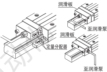
图1 结构图
