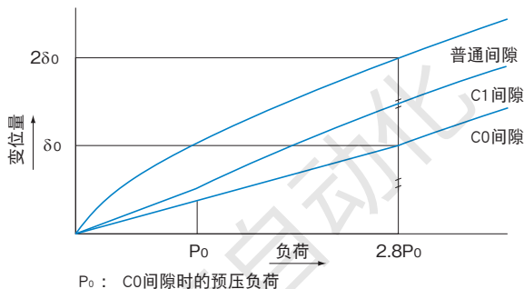
图10 刚性数据
