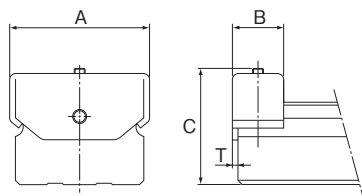
图1 NR/NRS型的末端止动块EP型
