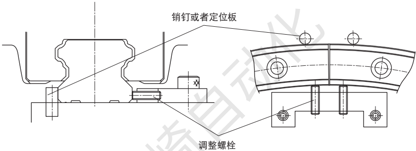
图7 押板固定
