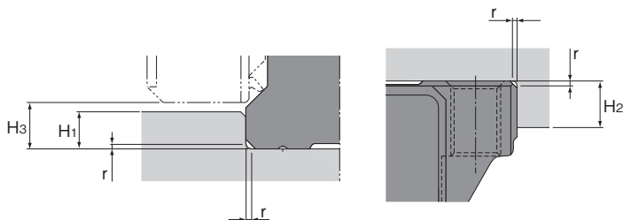
LM轨道的肩部
