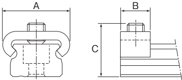
图1 RSR-Z/RSR-WZ型制动器(C型)
