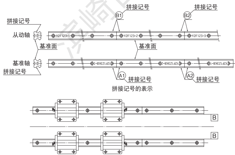
图23 拼接使用
