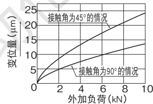
图2 径向载荷和变位置(通常间隙、无预压)
