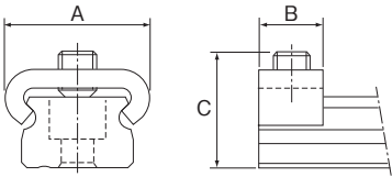
图1 RSR/RSR-W型制动器(C型)
