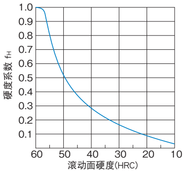
图8 硬度系数 (f H )
