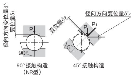
图1 径向载荷下的变位置
