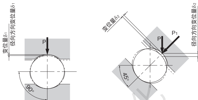
图3 径向载荷下的变位量
