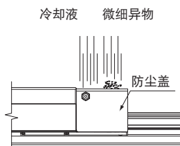
防尘盖内部构成图 (例：QZJJHH式样时)
