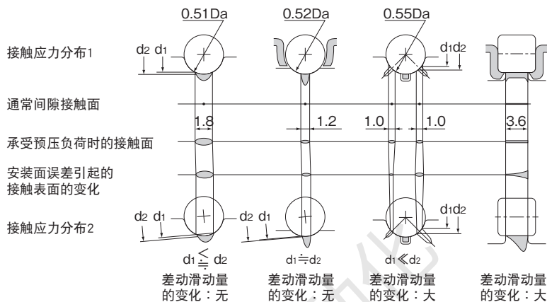
图4 接触面的比较( \phi 6.350钢球, \phi 6 \times 6 \ell 滚柱)
