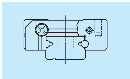
图 1 LU 系列
