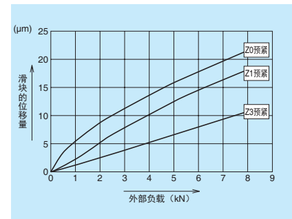
图 3.3 压缩方向的刚度 (SH35)
