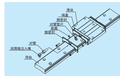
图 10 双密封
