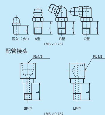
图 12 润滑脂注油孔和专用配管连接头
