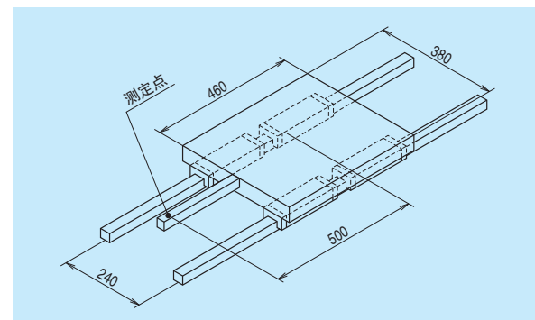
图 5 钢球通过震动测定概略图
