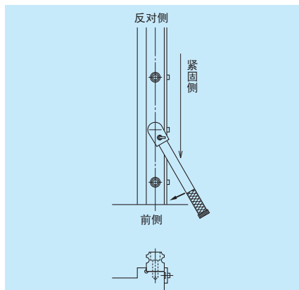
图 10.14 导轨的安装
