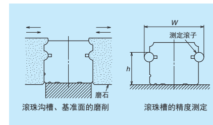
图 4 导轨磨削与测定
