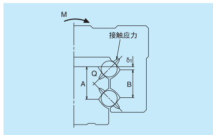
图 2 槽扩大图 (偏置哥特式弧状) 接触应力
