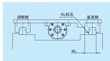
图 10.3 根据使用情况而采用的基准选取方法
