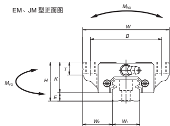
EM、JM 型正面图
