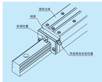
图 13 润滑用部件的安装位置
