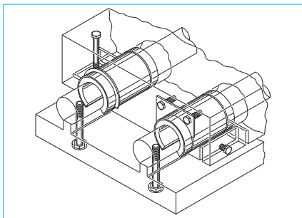
图 11 开放型的安装示例
