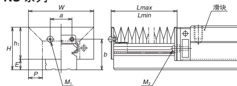
图 17 波纹管尺寸图
