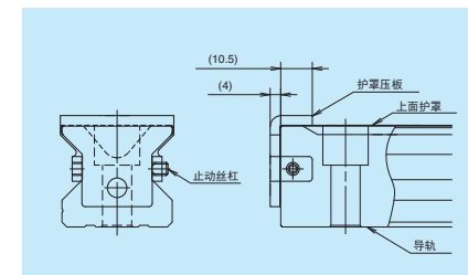
图 20 使用导轨上面护罩时的导轨端部
