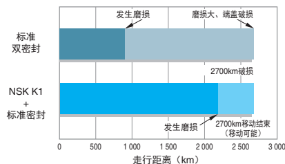
图 6.3 水没耐久试验结果
