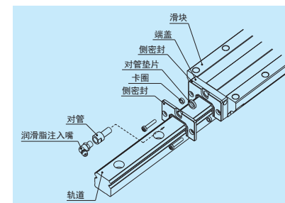
图 15 双密封
