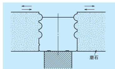
图 3 导轨研磨
