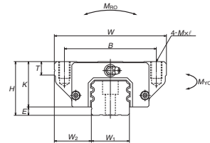
EL、GL 型正面图
