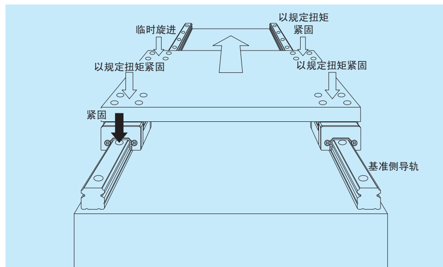
图 10.18 简单安装
