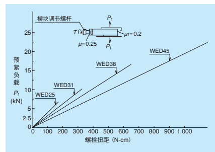
图 5 调节螺杆的拧紧扭矩和预紧负载
