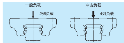
图 3 负载状态
