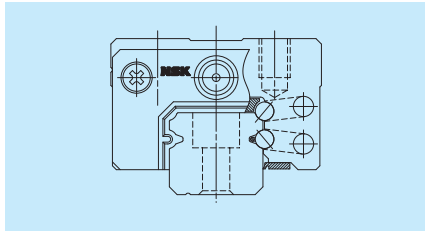
图 1 LH 系列
