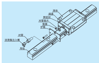
图 15 护板
