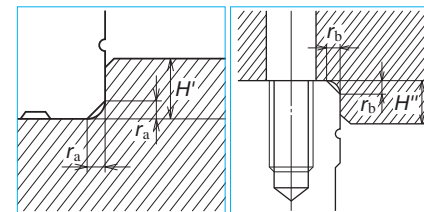
图 10.10 导轨基准面安装
