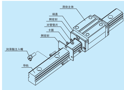
图 14 护板
