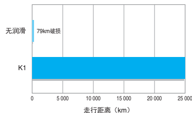
图 6.2 无润滑的耐久实验结果
