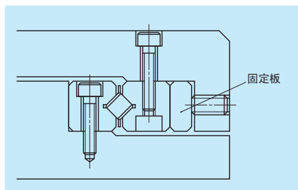
图 12 用垫板固定的示例
