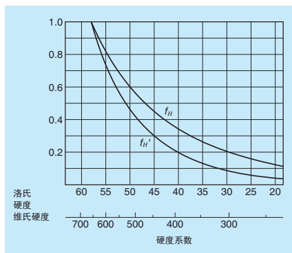
图 2.6 硬度系数
