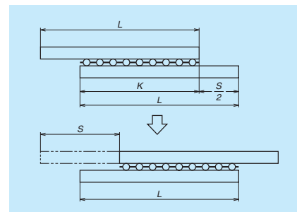
图 9 导轨和保持架的关系
