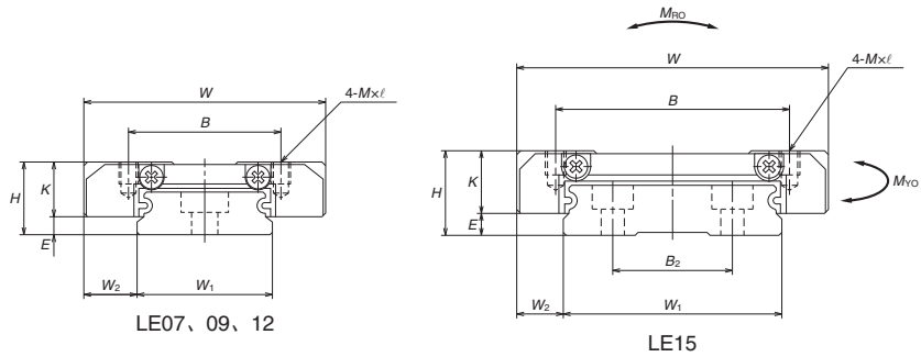
正面图
