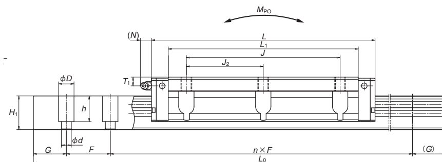
EM 型侧面图
