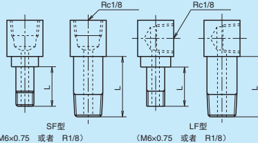
图 14 润滑脂注入嘴和专用配管接头
