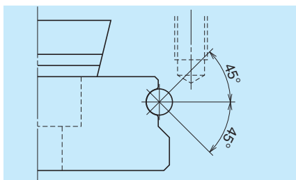
图 2 滚珠接触状态
