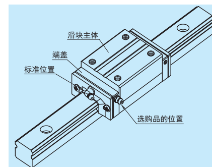
图 13 润滑用零件的安装位置
