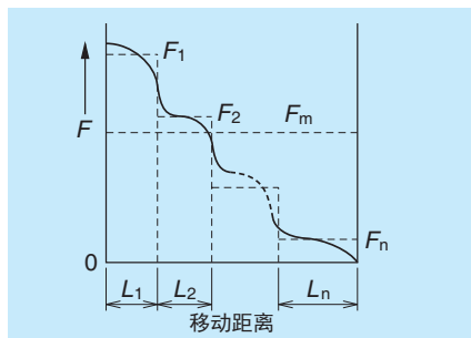
图 2.3 阶段性变动负载
