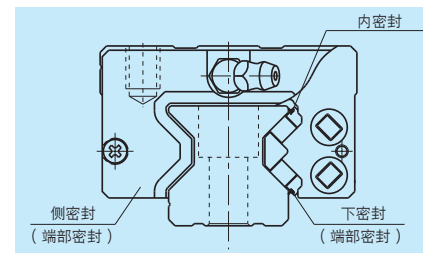
图 15
