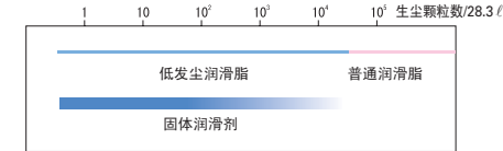
图 9.2 清洁环境下的润滑
