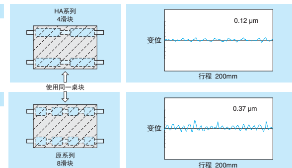
图 6 HA 系列与先前系列的测定结果
