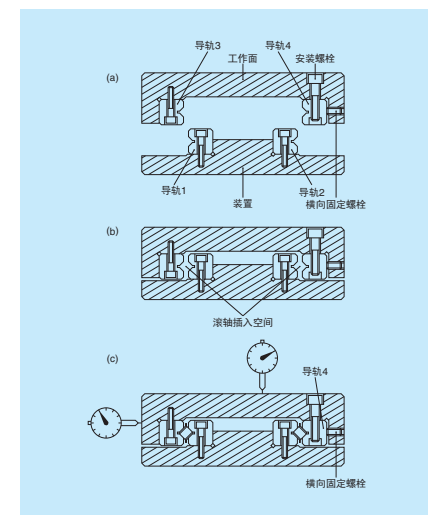
图 11 标准安装顺序
