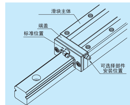
图 13 润滑零件的安装位置
