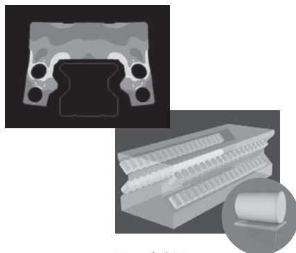
图 2 解析图
