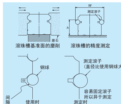
图4 沟槽的加工与测定
