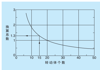
图 7 弹性变形量的换算系数
