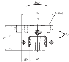
AN、BN 型正面图
