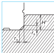
图 5 导轨基准面安装部
