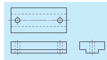
图2 装配板
