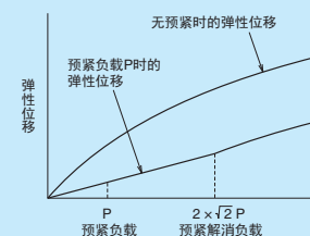
图 3.2 弹性位移曲线
