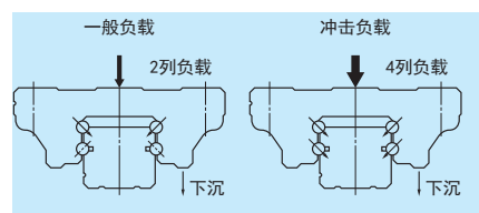
图5 抗冲击性
