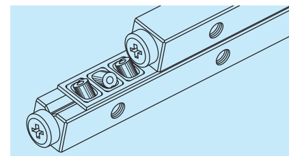
图 1 叉滚子导轨的结构
