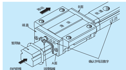
图 10.23 互换性滑块插入导轨中
