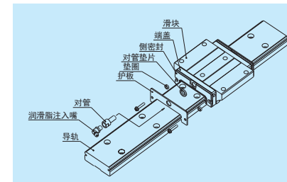
图 11 护板
