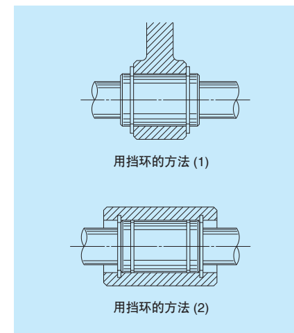
图 9 用挡环的安装
