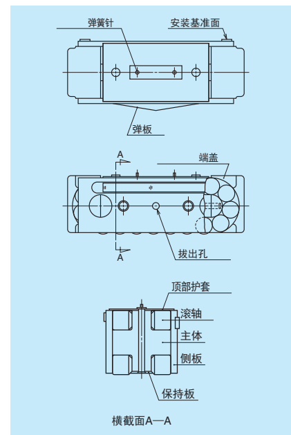
图1 滚子组件
