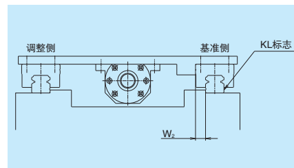
图 10.2 常用基准的选取方法
