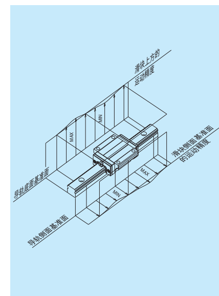
图 4.2 走行平行度
