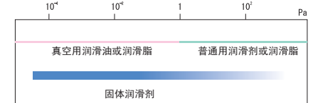
图 9.3 真空环境下的润滑
