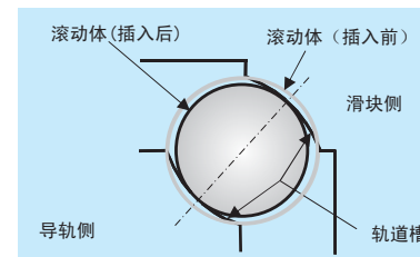
图 3.1 预紧方法
