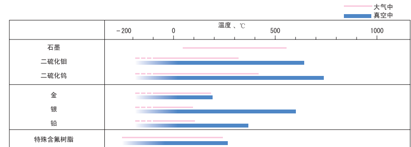
图 9.8 固体润滑剂使用温度范围
