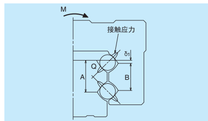
图 2 沟槽放大图 (偏移哥特式圆弧)
