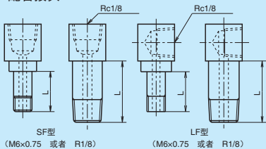
图 11 润滑脂注入嘴和专用配管接头
