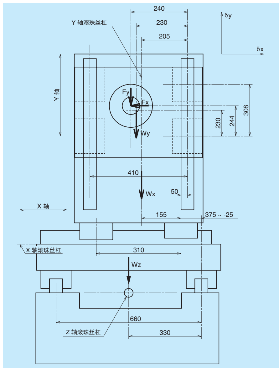
图 11.2 加工中心（正面图）
