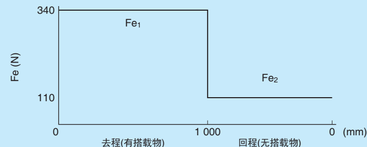
全动态等效负载循环模型
