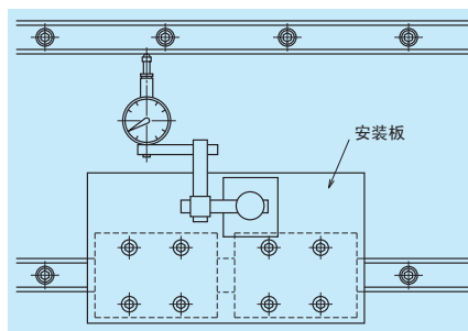
图 10.15 平行度测试
