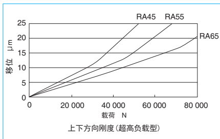
图7 上下方向理论刚度线图：超高负载型（滑块形状：BN、BL、GM）
