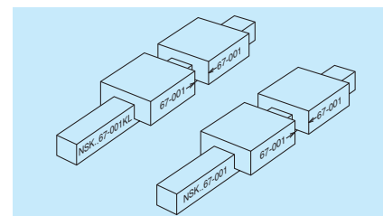
图 10.30 2根导轨公称型号不同时
