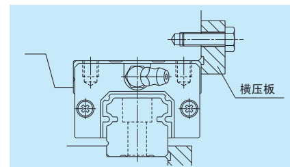
图 10.17 滑块横压
