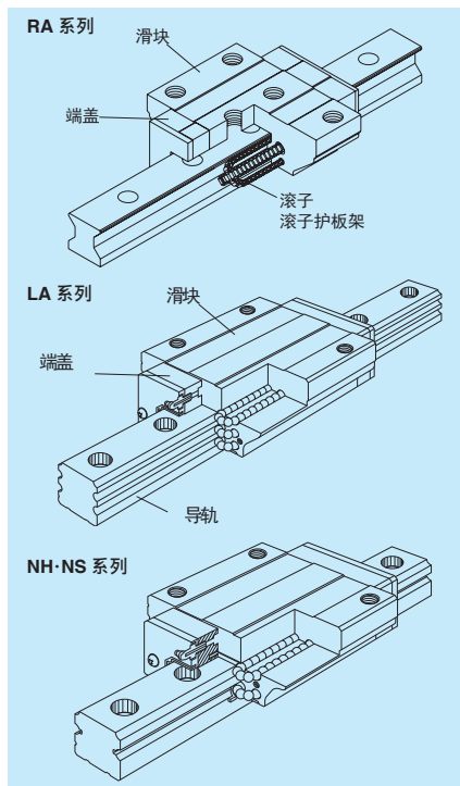
图2 NSK直线导轨的结构
