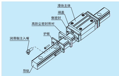
图 15 双密封
