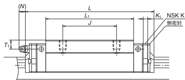
BN 型侧面图
