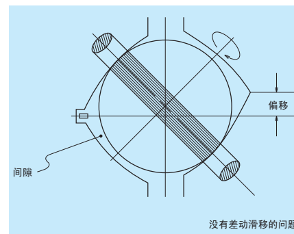
图3 依靠偏移哥特式圆弧沟槽的2点接触
