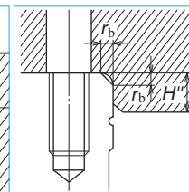
图 10.11 滑块基准面安装部
