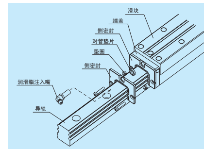
图 15 双密封
