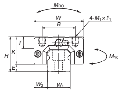
AL、BL 型正面图
