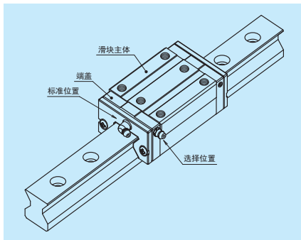
图 12 润滑用零件的安装位置
