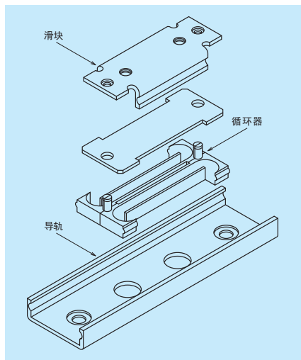
图 1 LL 系列构造
