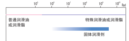
图 9.7 放射线环境下的润滑
