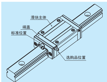
图 12 润滑用零件安装位置
