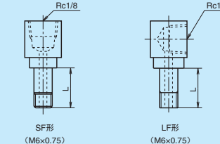
图 1 润滑脂注入嘴和专用配管接头
