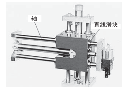
图 8 安装例
