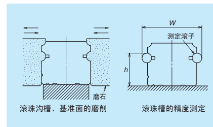
图 4 导轨磨削与测量
