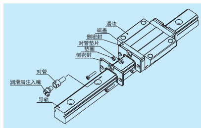
图 14 双密封
