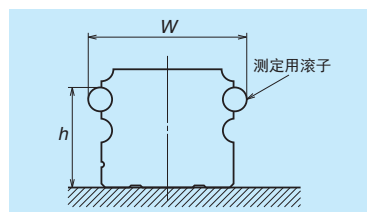
图 4 沟槽的精度测定
