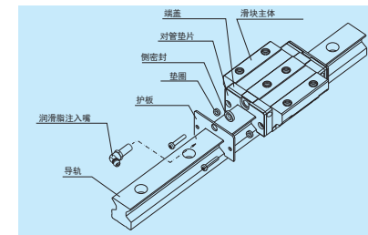
图 18 护板
