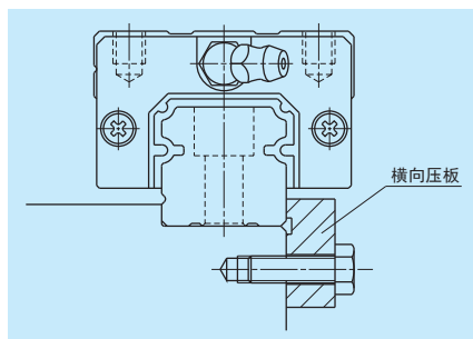
图 10.13 导轨横向加压
