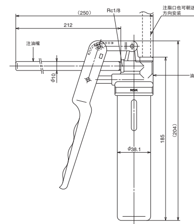
图 6.7 带 NSK 直接注油嘴的 NSK 手持式润滑脂枪
