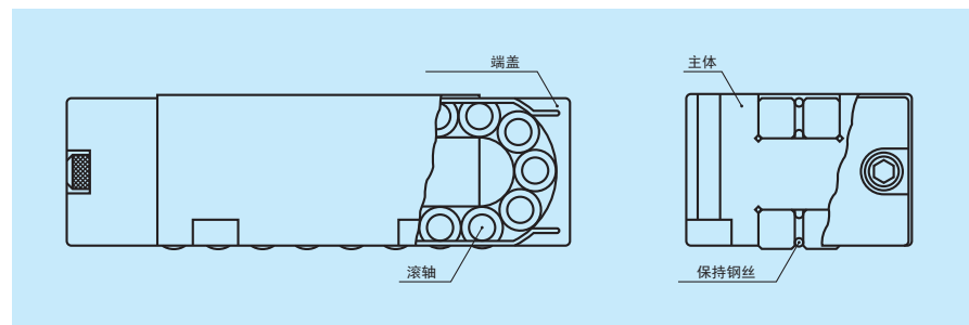
图 1 直线滚子轴承
