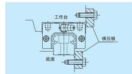
图 10.19 推荐图
