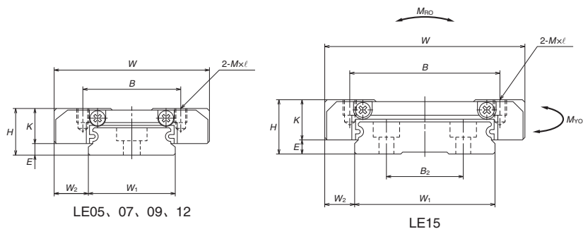
正面图
