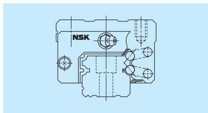
图 1 NH 系列
