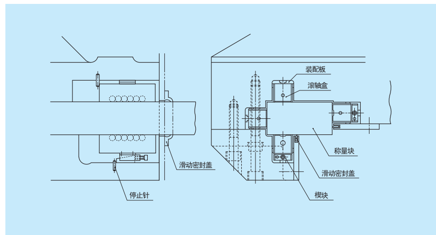
图 7 滚子组件包装箱的设计示例
