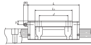
FL 型侧面图
