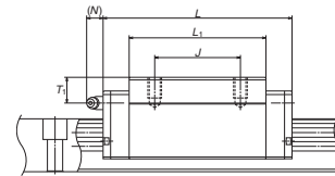
AN 型侧面图
