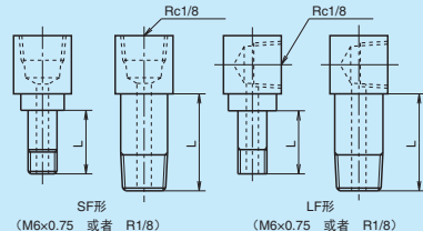
图 7 润滑脂注入嘴和专用配管接头
