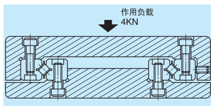
图 8 弹性变形量的计算例、图
