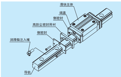
图 16 护板
