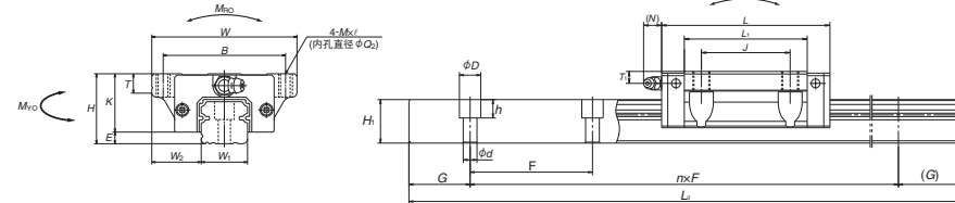
EM、GM 型正面图
