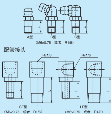
图 10 润滑脂注入嘴和专用配管接头
