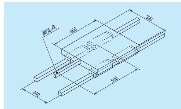
图 5 钢球通过振动测定概略图
