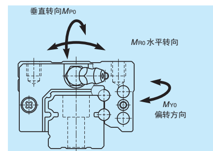
图 2.8 扭矩负载的方向
