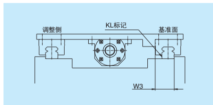
图 4.4 组装宽度尺寸 W_3
