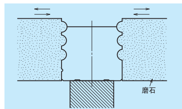
图 3 导轨磨削
