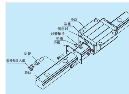
图 7.3 护板
