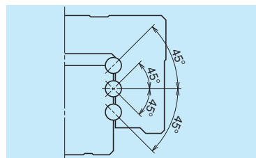
图 2 超高刚度设计
