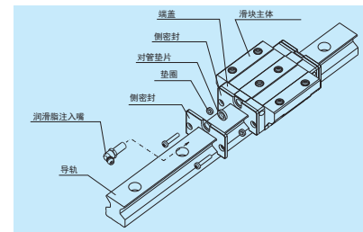
图 17 双密封
