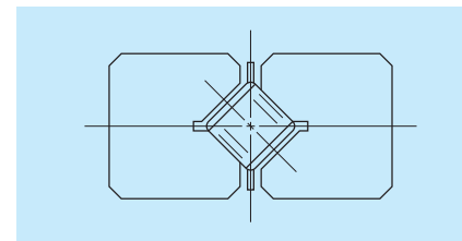
图 2 交叉滚子导轨的剖面图
