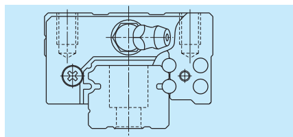
图 1 HS 系列
