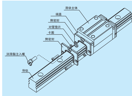
图 13 双密封
