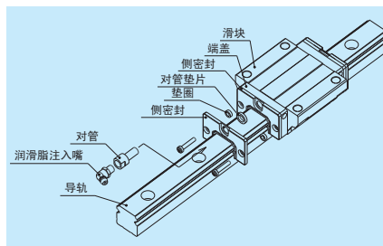
图 7.2 双密封
