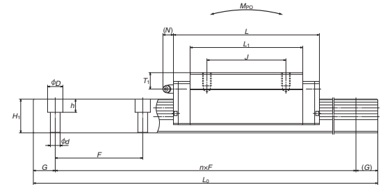
BN 型侧面图
