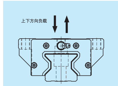
图 5 负载的方向
