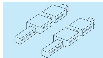
图 10.29 2根导轨公称型号相同时
