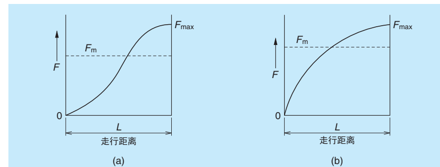
图 2.5 按正弦曲线变化的负载
