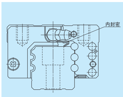
图 7.6 内密封安装状况
