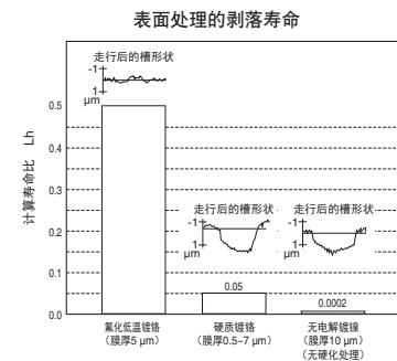
图 8.1 耐久试验结果
