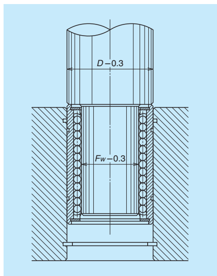
图 10 直线滚珠滑块的安装工具示例
