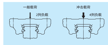
图 3 负载状态
