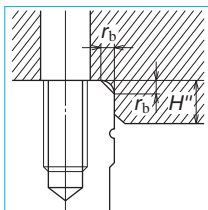
图 6 滑块基准面安装部
