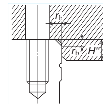
图 10 滑块基准面安装部
