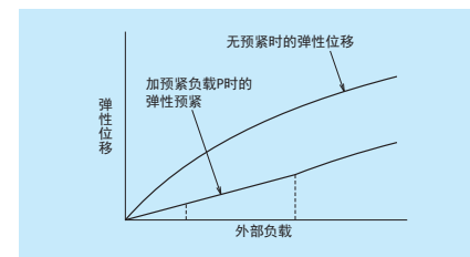
图 3.9 弹性位移曲线
