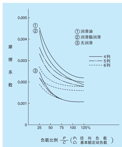
图 4 直线滚珠轴承的动态摩擦系数
