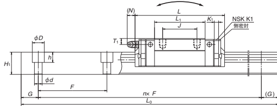
AL 型侧面图
