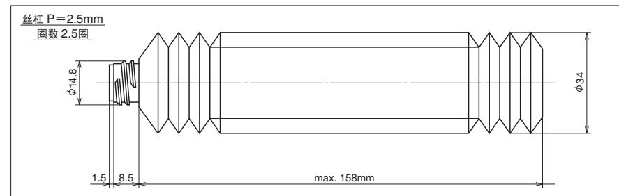
图 6.6 波纹容器
