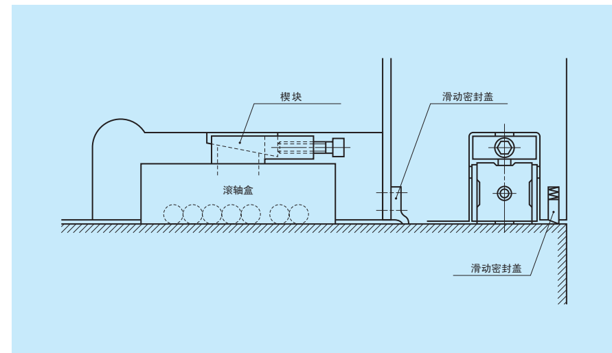
图 6 密封方法
