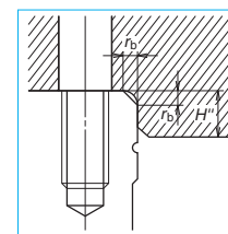
图11 滑块基准面安装部
