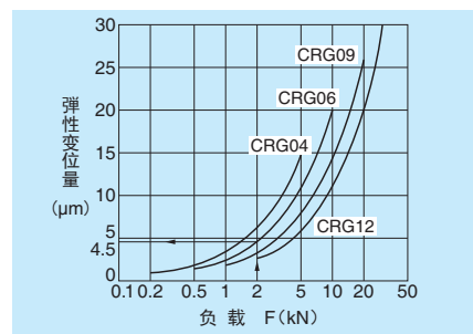
图 6 20 个滚子时的弹性变形量
