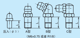
配管接头
