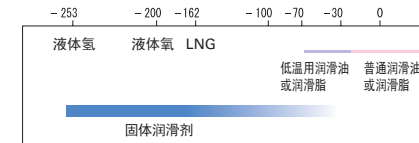
图 9.6 低温环境下的润滑
