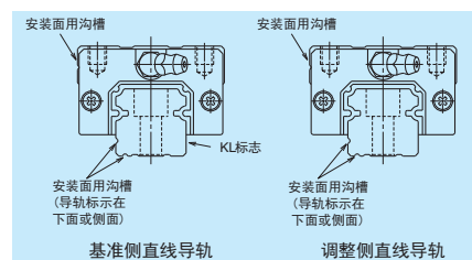
图 10.1 基准面
