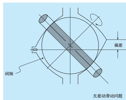
图3 偏移哥特式沟槽的2点接
