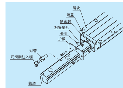
图 16 护板
