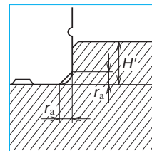
图 9 导轨基准面安装部
