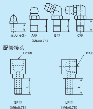
图 11 润滑注入嘴和专用配管接头
