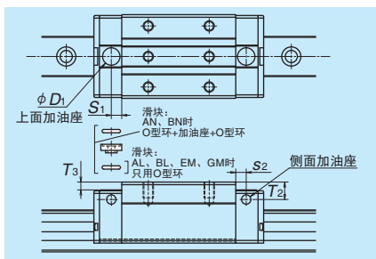
图 13 侧面、上面加油孔位置
