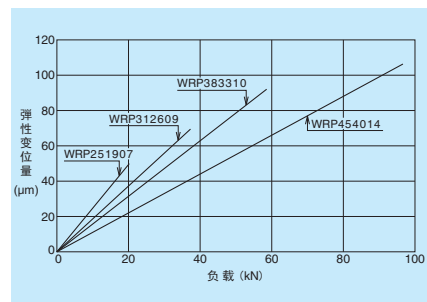
图 4 滚子组件弹性变形量
