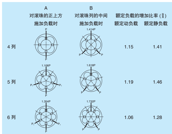
图 7 根据滚珠列位置的额定负载增加率 (B/A)
