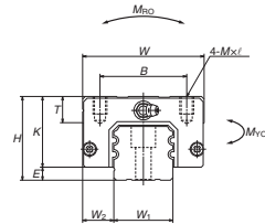
AL、BL 型正面图
