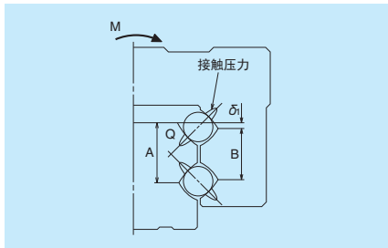
图 2 沟槽放大图 (偏移哥特式圆弧)
