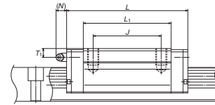
EL 型侧面图
