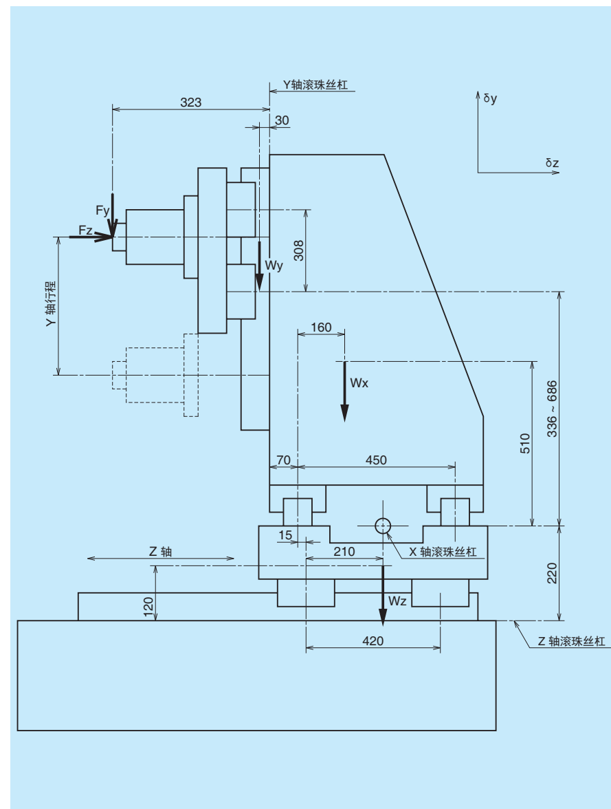
图 11.3 机械加工中心（侧面图）
