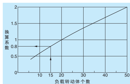
图 13 基本额定静负载的换算系数
