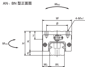
AN、BN 型正面图
