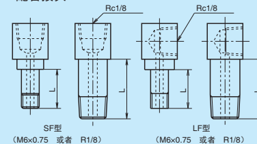
图 12 润滑脂注入嘴与专用配管接头
