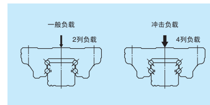
图 3 负载状态
