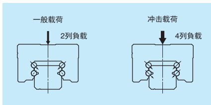
图 3 负载状态
