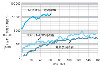
图 6.5 产尘特性的比较
