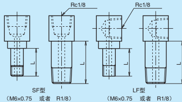
图 12 润滑脂注油孔和专用配管接头
