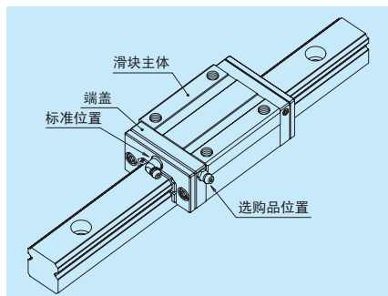
图 12 润滑用零件的安装位置
