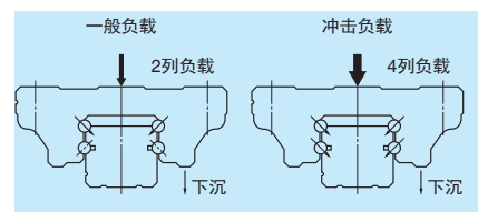
图5 耐冲击性
