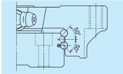
图 1 滚珠接触状态
