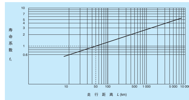
图 5 寿命系数与行走距离的关系
