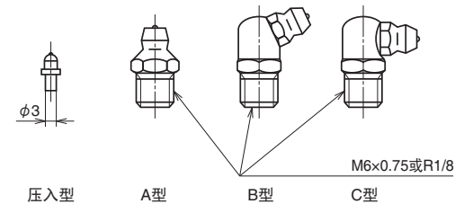
图 6.8 润滑脂注入口形状
