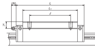
BN 型侧面图
