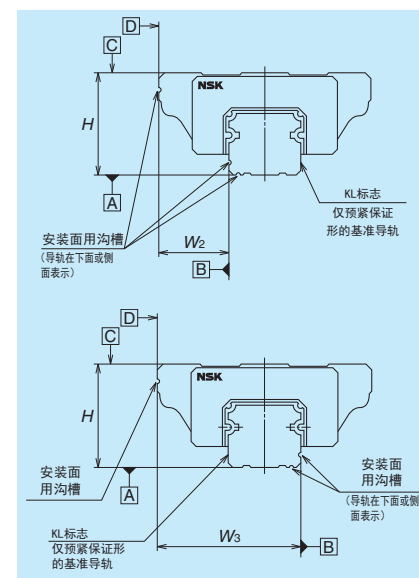
图 4.1 组装尺寸
