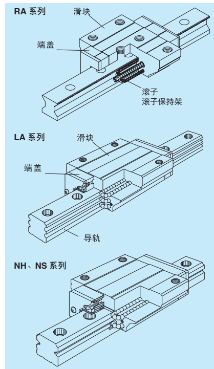
图2 NSK直线导轨的结构
