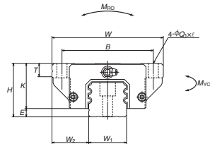
FL、HL 型正面图
