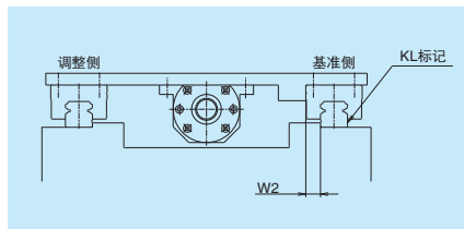
图 4.3 组装宽度尺寸 W_2
