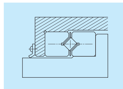
图 10 防尘示例
