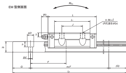
JM 型侧面图
