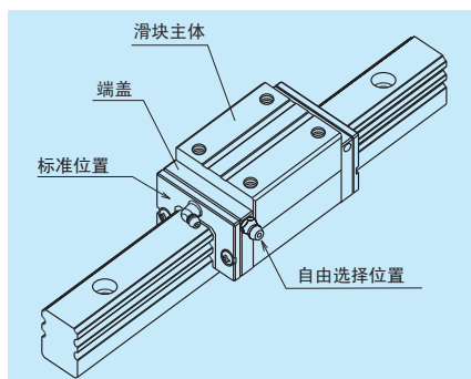
图 11 润滑零件的安装位置
