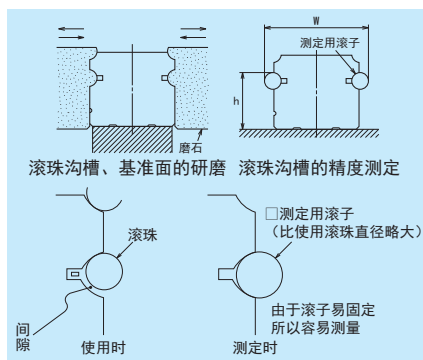
图4 沟槽的加工和测定
