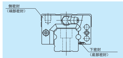
图 1 VH 系列
