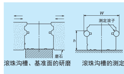
图 4 导轨研削和测量
