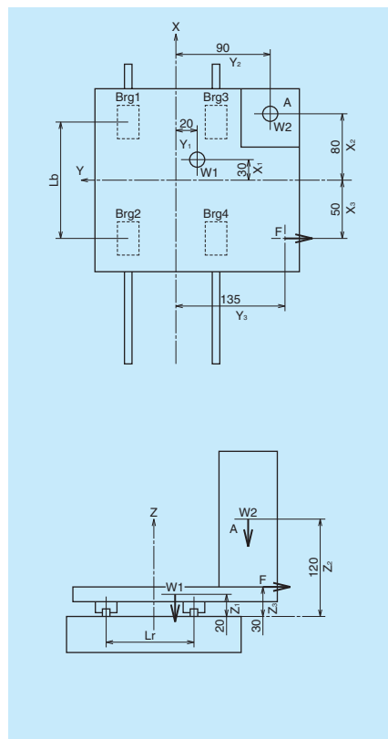
图 11.1 单轴搬运装置
