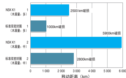
图 6.4 木屑耐久试验结果
