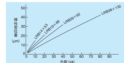
图 2 弹性变形量
