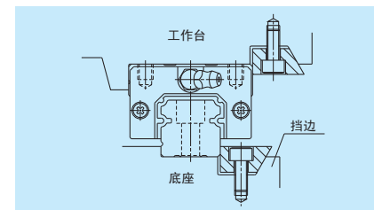
图 10.20 应注意的安装
