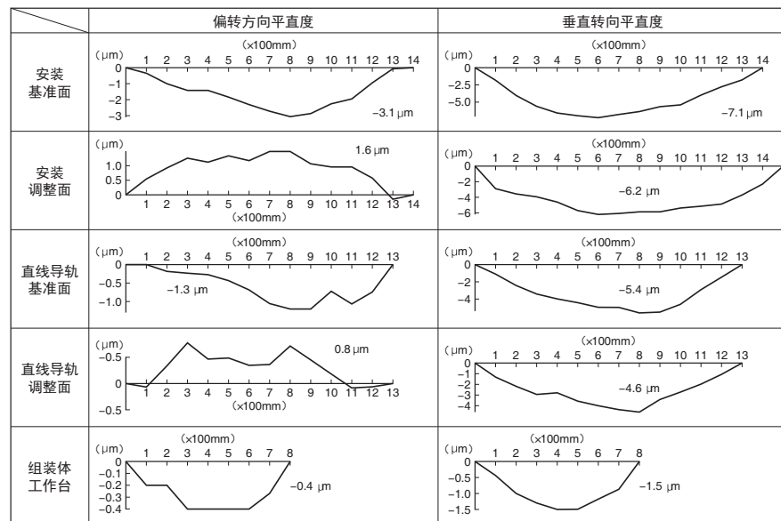
图 10.9 采用直线导轨的工作台平直度
