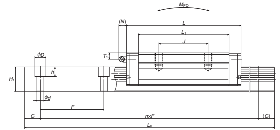
GL 型侧面图
