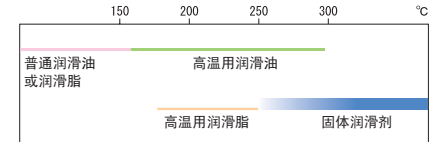
图 9.5 高温环境下的润滑
