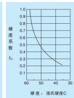
图 6 硬度系数
