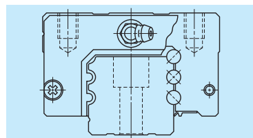
图 1 LA 系列
