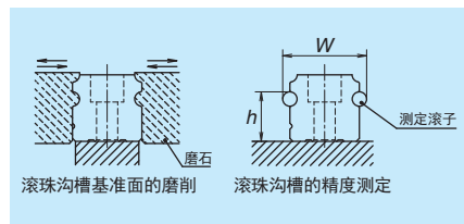
图 4 导轨磨削与测量
