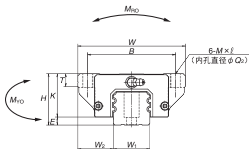
EM 型正面图
