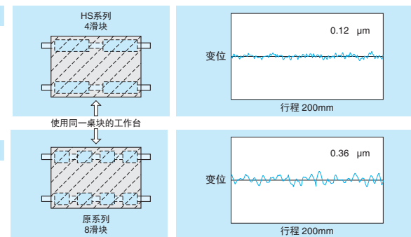
图 6 HS 系列和先前系列的测定结果
