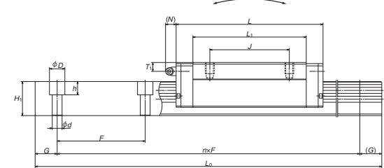
BL 型侧面图
