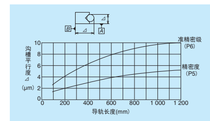
图 3 滚子行走面的平行度
