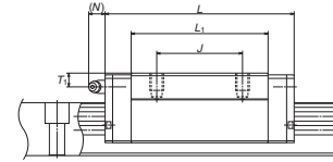
AL 型侧面图
